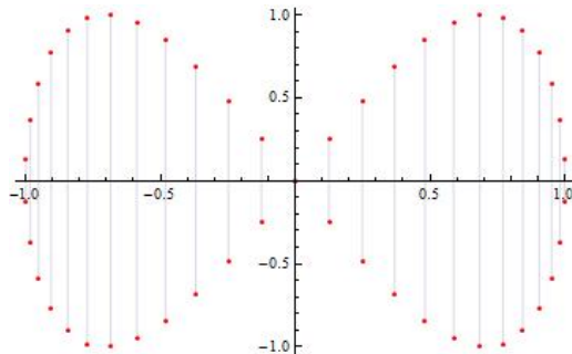
Kuva 1: Geronon lemniskaatta välillä [-1, 1] .
